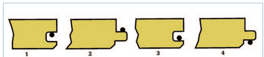
Figur 6. Limpåføringsmetoder ved flytende parkett.
