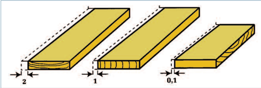
Figur 5. Fuktbevegelser for trevirke.
